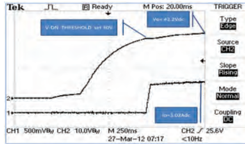
Fig. 3 eLOAD Scope Trace
